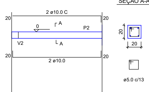
SEÇÃO A-A
