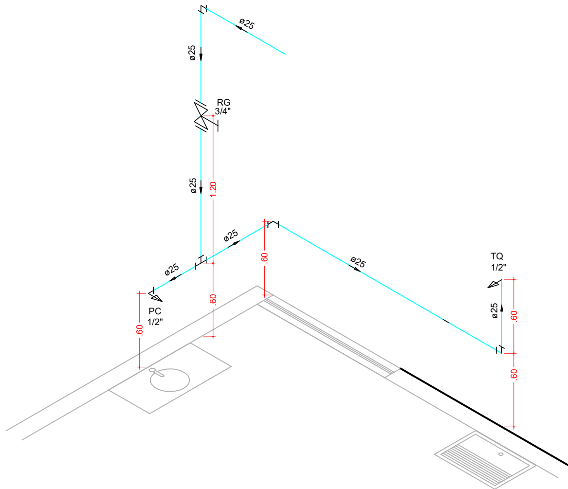
DETALHE H2 Esc.: 1/30
