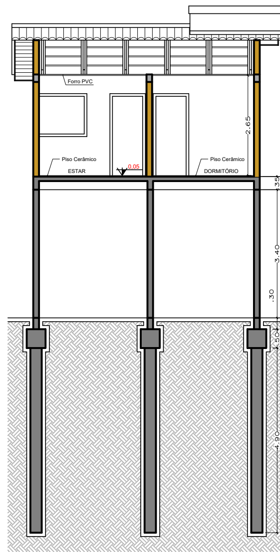
CORTE AA' Esc.: 1/100
