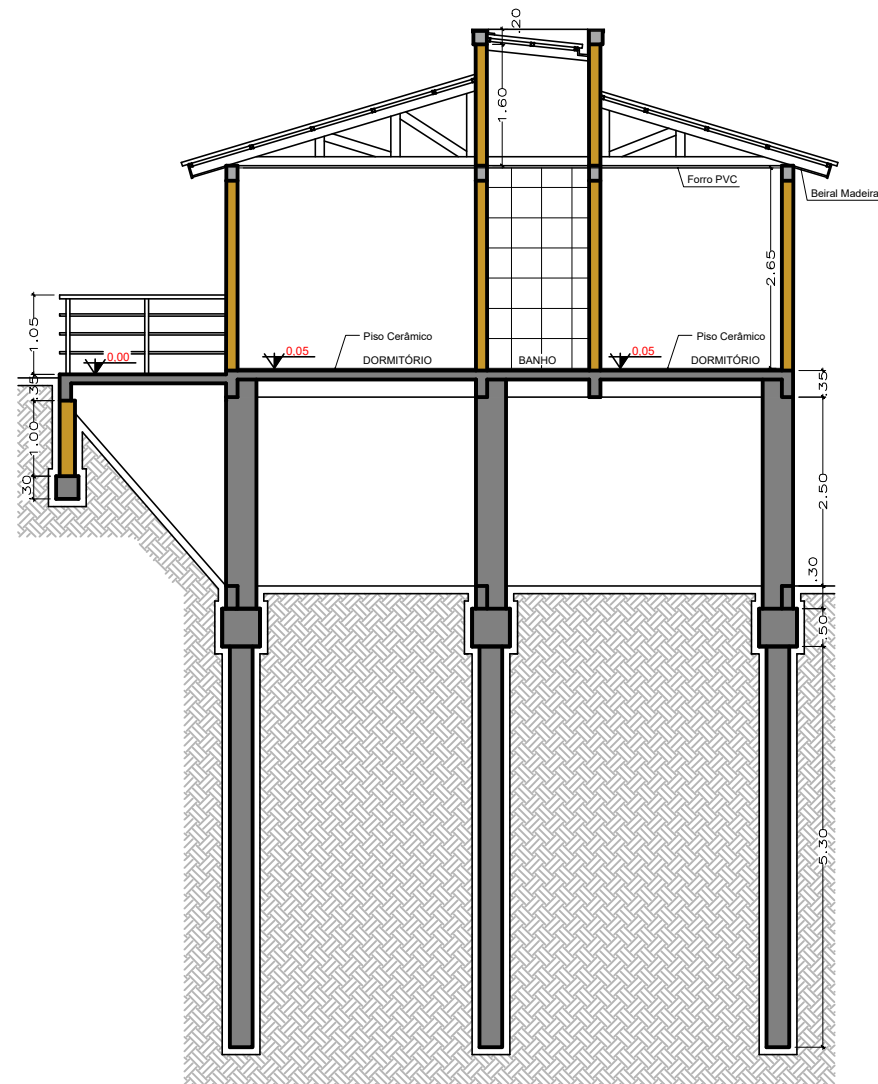
CORTE BB' Esc.: 1/100
