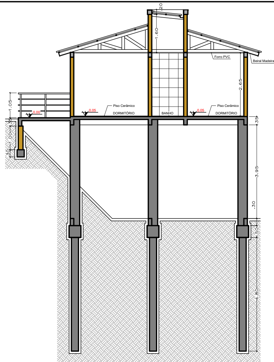
CORTE BB' Esc.: 1/100
