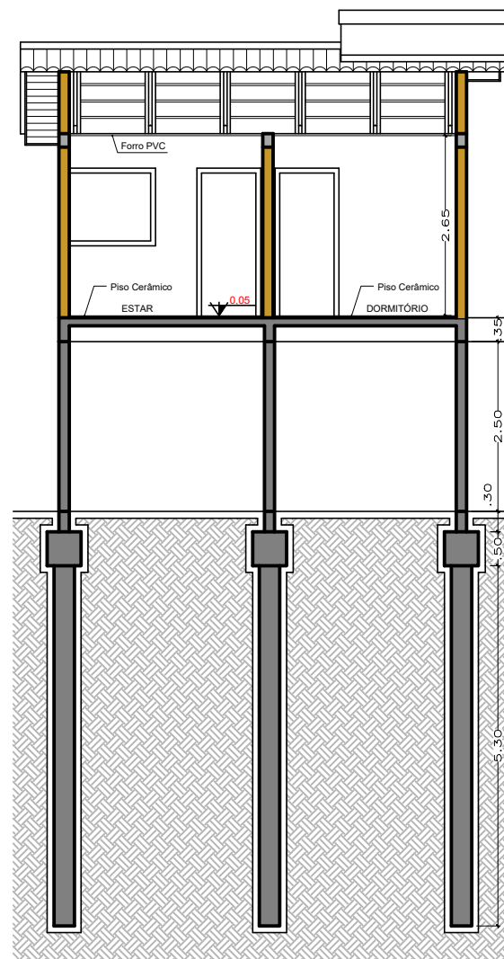
CORTE AA' Esc.: 1/100
