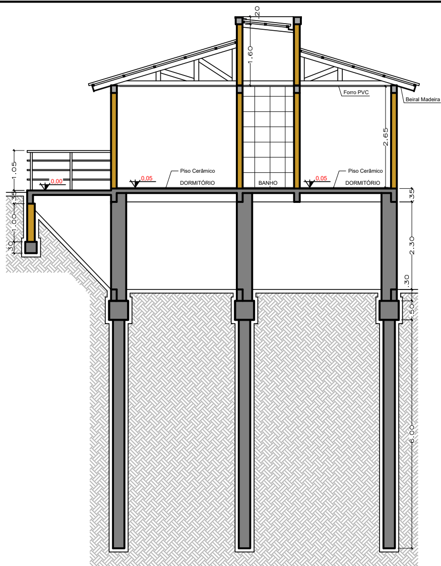
CORTE BB' Esc.: 1/100
