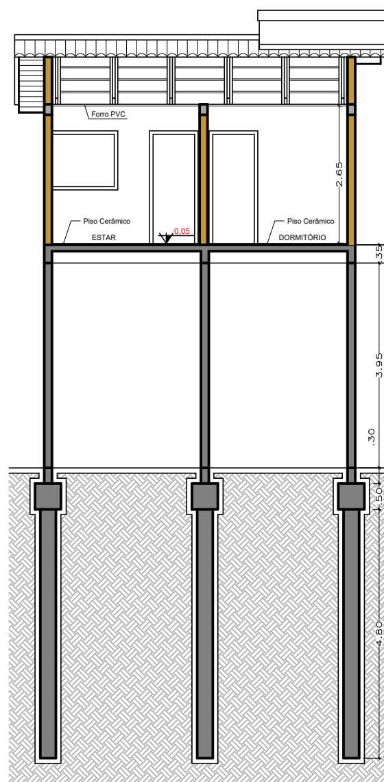
CORTE AA' Esc.: 1/100
