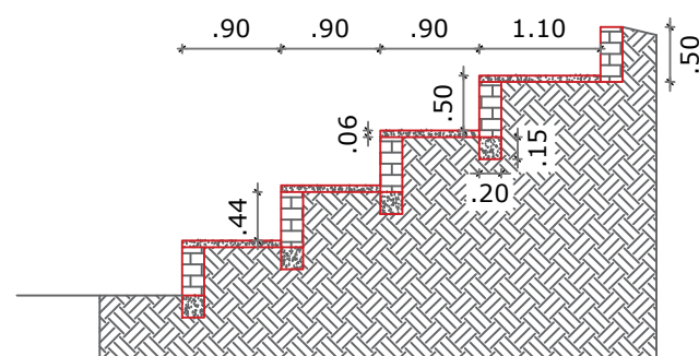
Corte lateral
