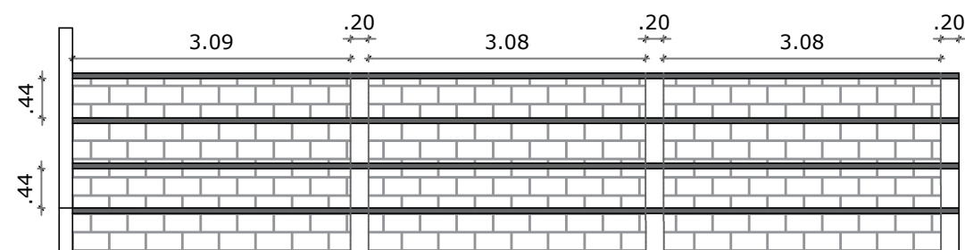
Corte frontal
