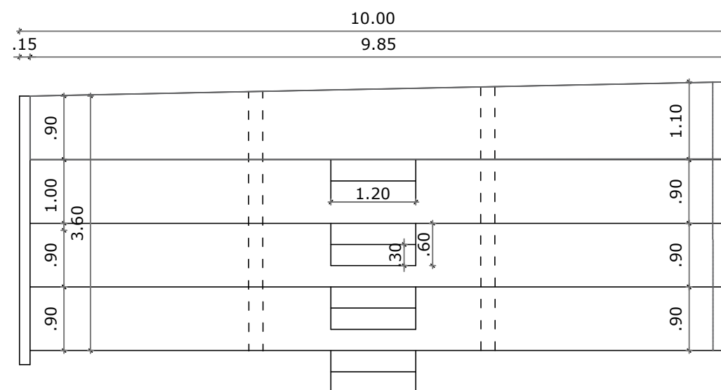
Planta Baixa
