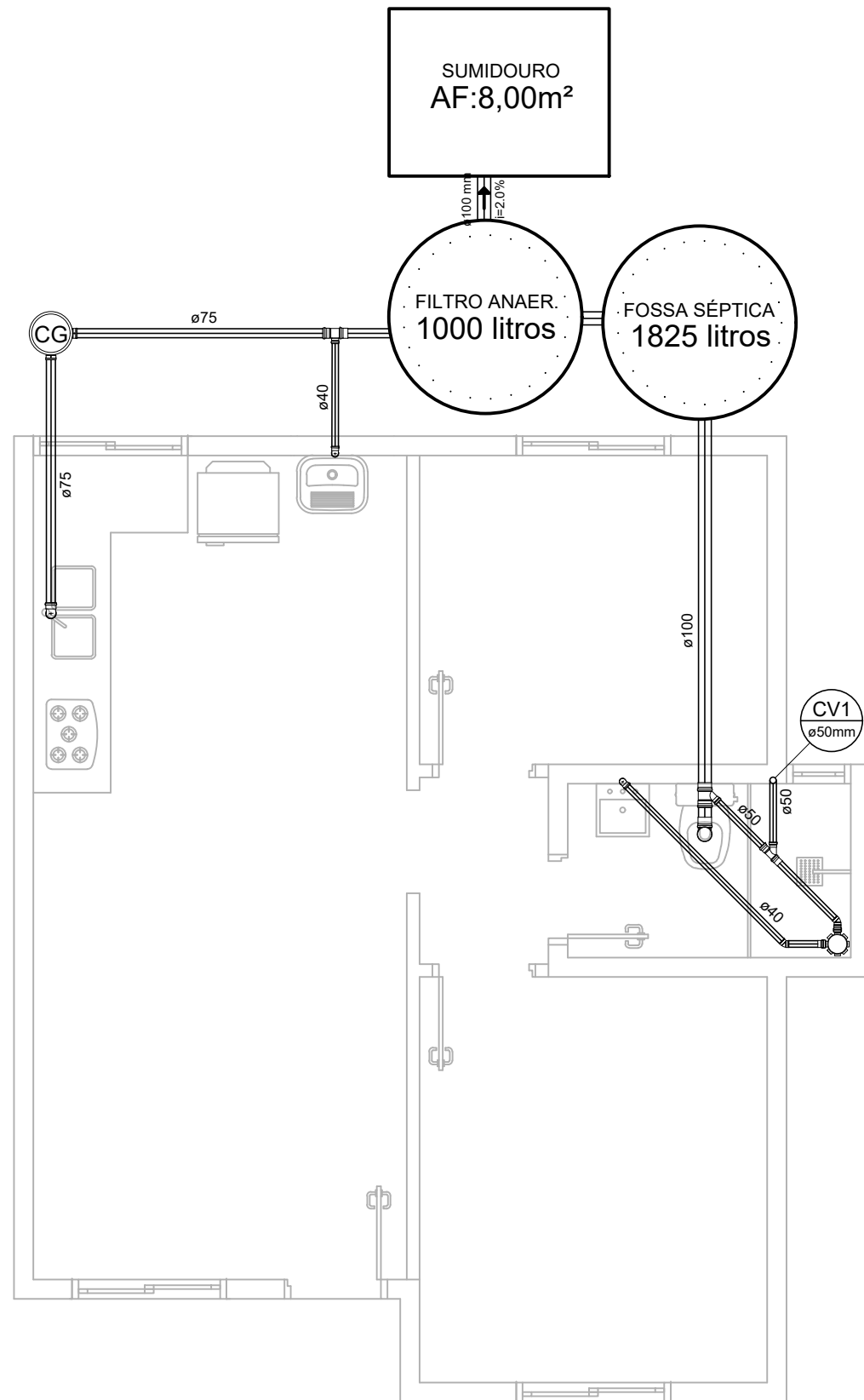
PLANTA BAIXA INST. SANITÁRIAS Esc.: 1/50
