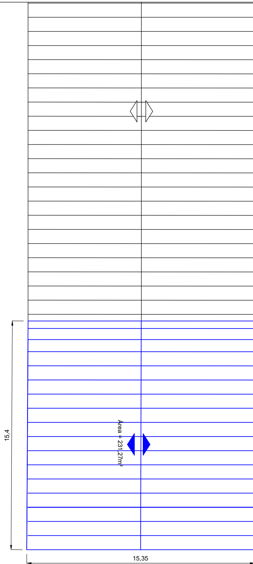
PLANTA DE COBERTURA Esc.: 1:150
