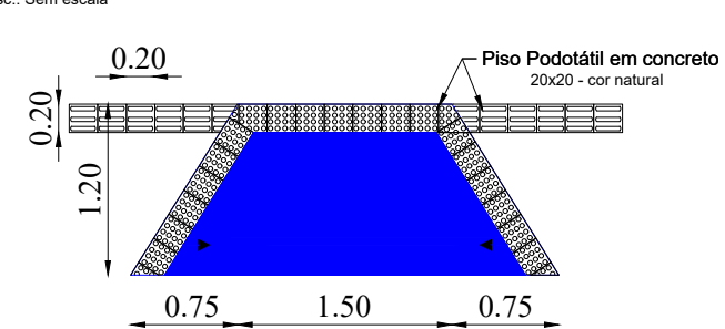
Detalhe 01 - Rampa para Faixa de Pedestre Esc.: Sem escala
