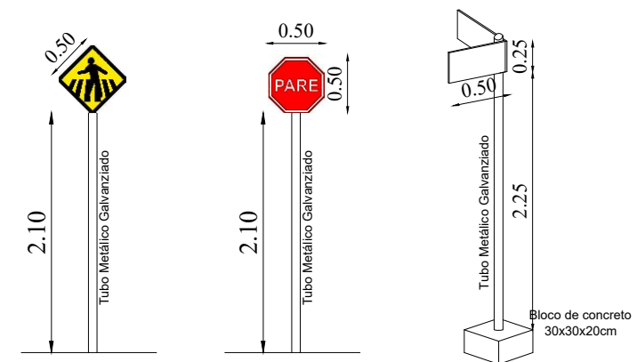
Detalhe 03 - Sinalização Vertical Esc.: Sem escala
