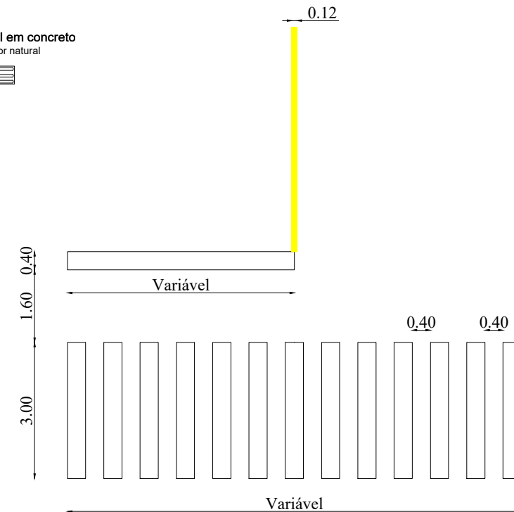
Detalhe 02 - Faixa de Pedestre Esc.: Sem escala
