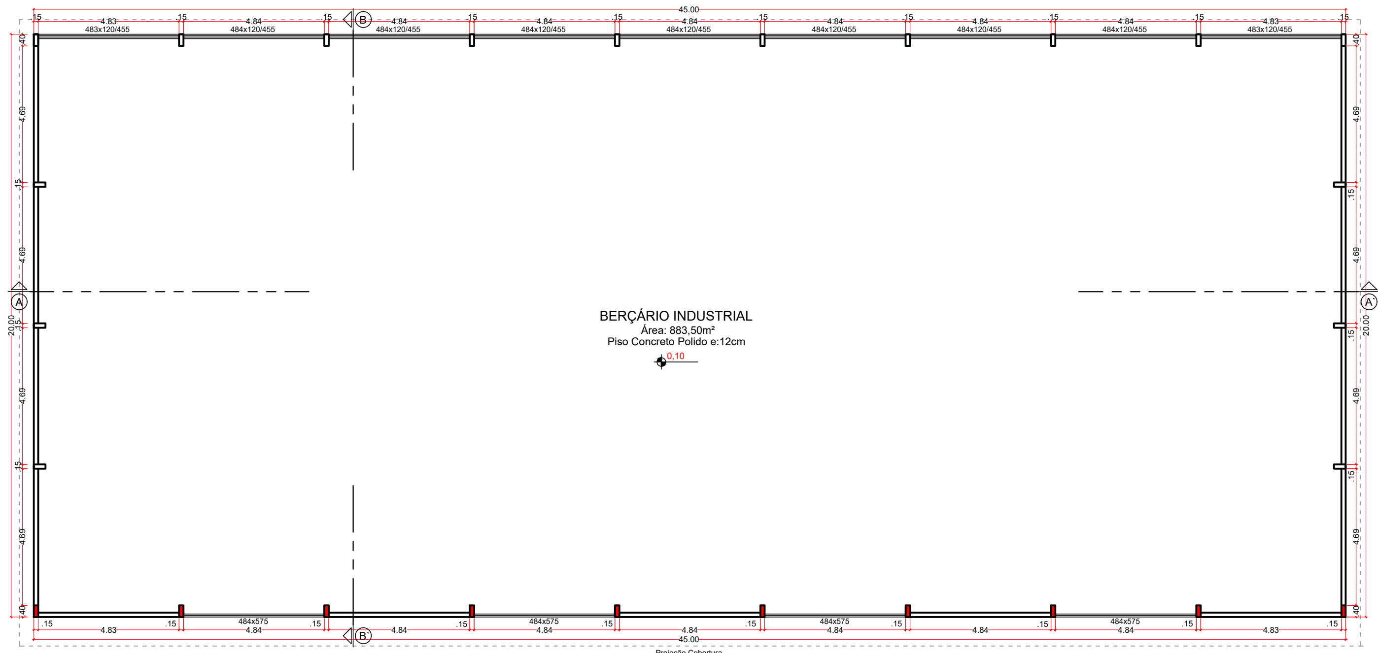
PLANTA BAIXA Esc.: 1/125 Área de construção: 900,00m²
