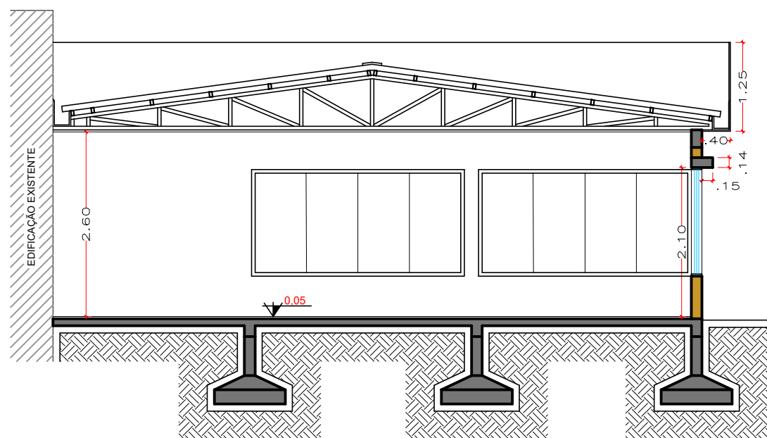
CORTE BB' Esc.: 1/75
