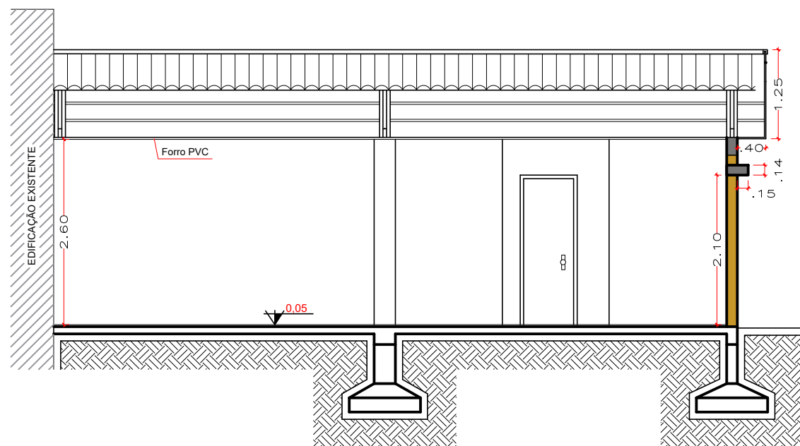
CORTE AA' Esc.: 1/75
