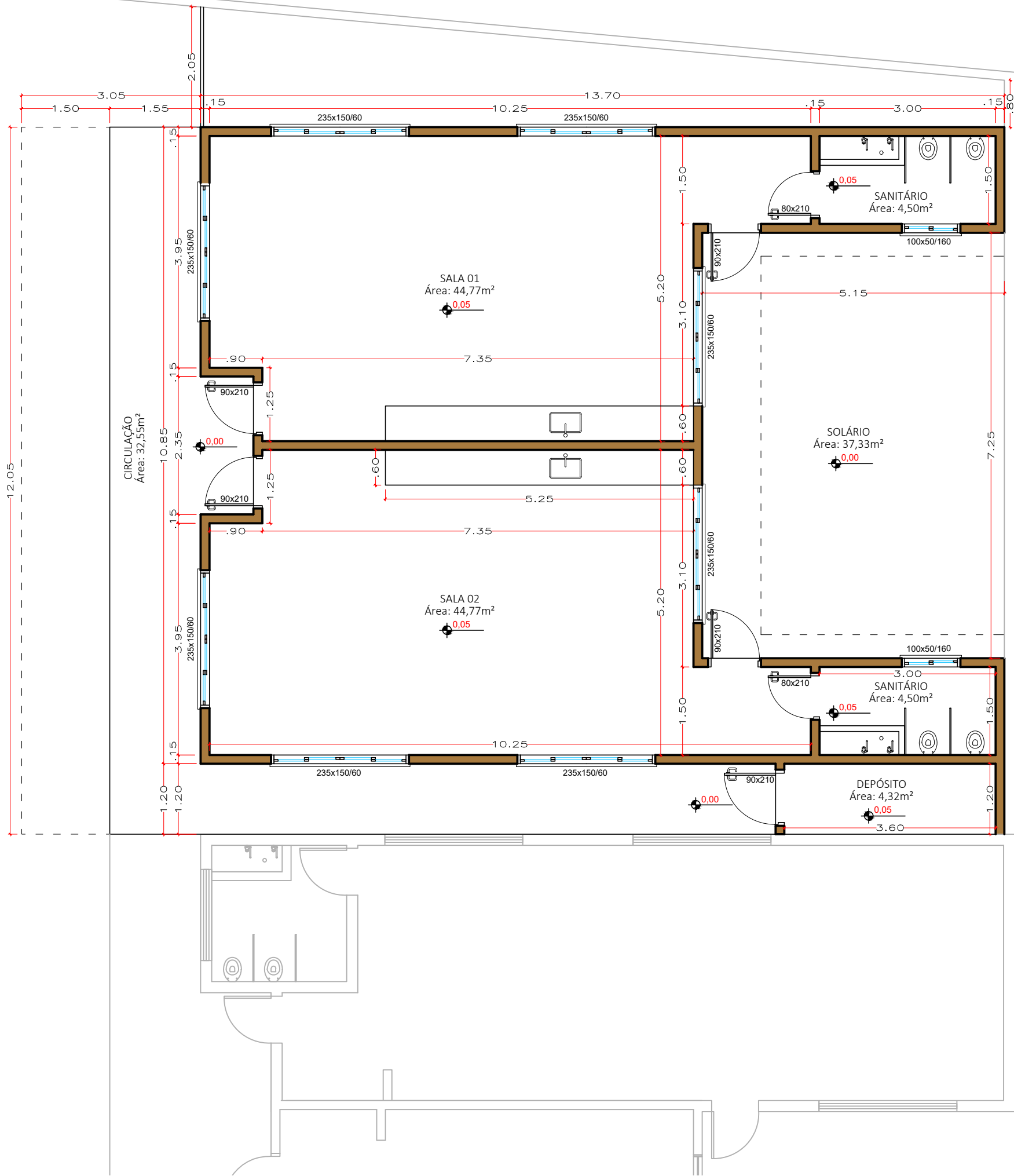
PLANTA BAIXA SALAS DE AULA Esc.: 1/75
